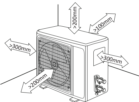
Esquema dimensional para instalação
