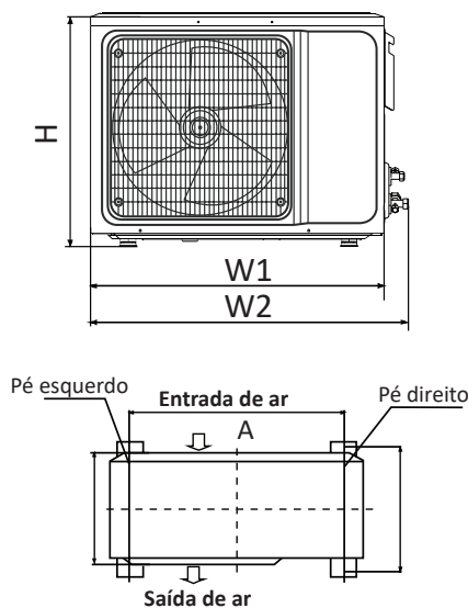
Dimensões da unidade exterior
